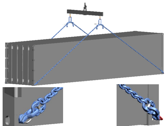
Container hook left hand „LH“
