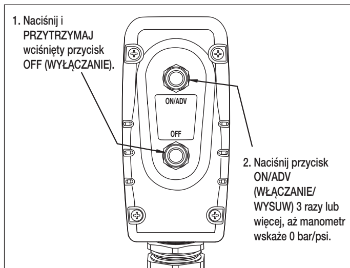
Rysunek 7, Redukcja ciśnienia (za pomocą przycisków kasety sterowniczej)
