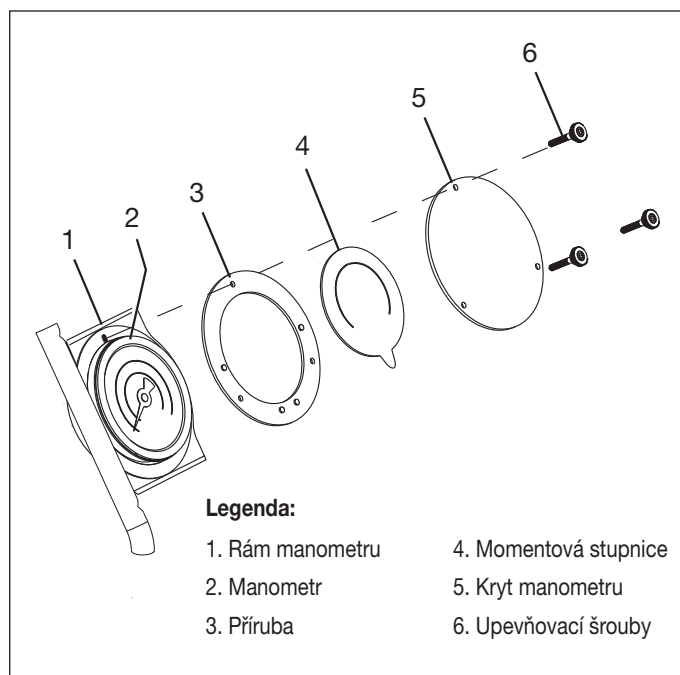
Obrázek 9, Momentová stupnice manometru
