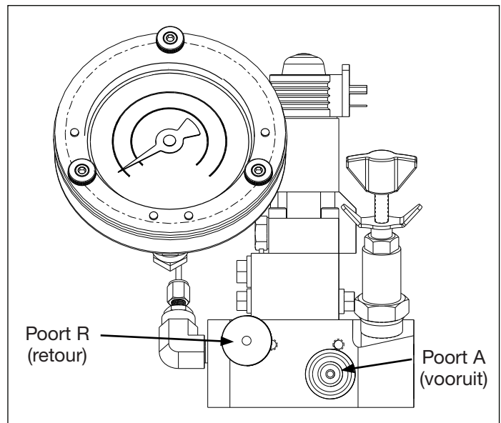
Figuur 4, Stuurventielpoorten
