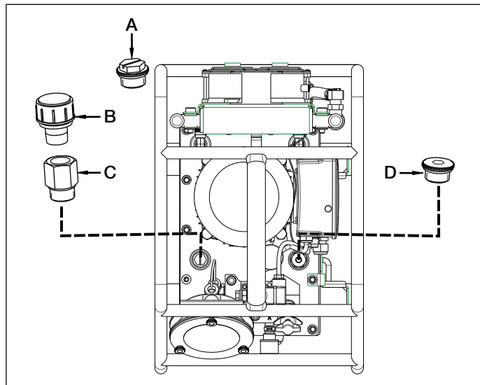
Obrázek 1, Odvzdušňovací ventil a zátka plnicího otvoru
