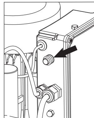
Rysunek 11, Wyłącznik ochronny obwodu
