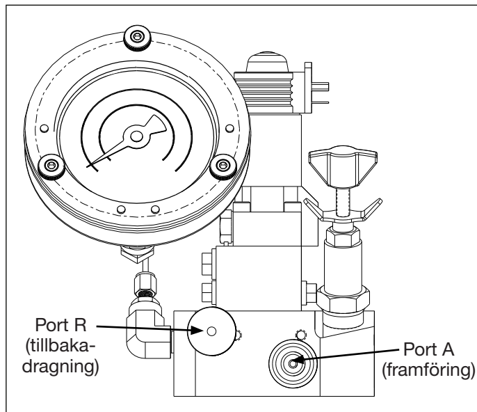
Figur 4, Ventilanslutningar
