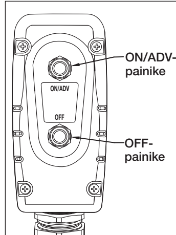
Kuva 6: Riippuohjaimen painikkeet
