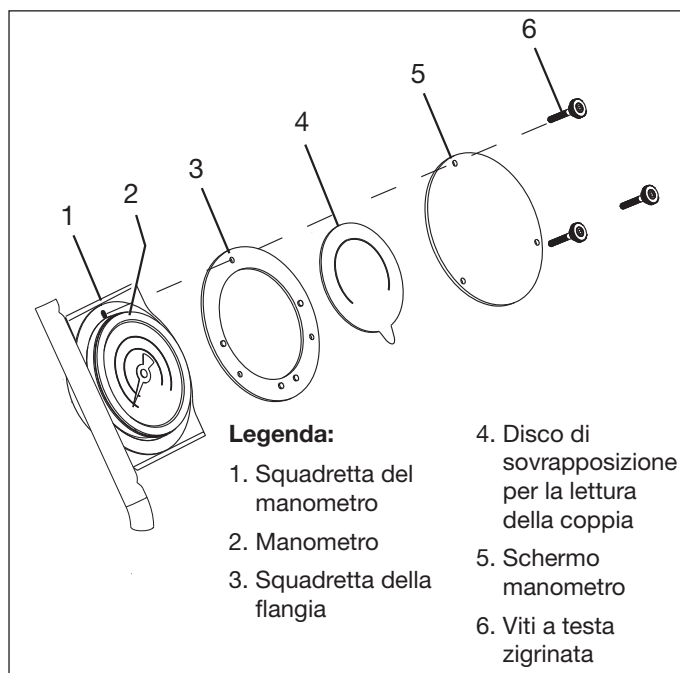
Figura 9, Disco di sovrapposizione manometro
