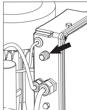
illustration 11, Disjoncteur
