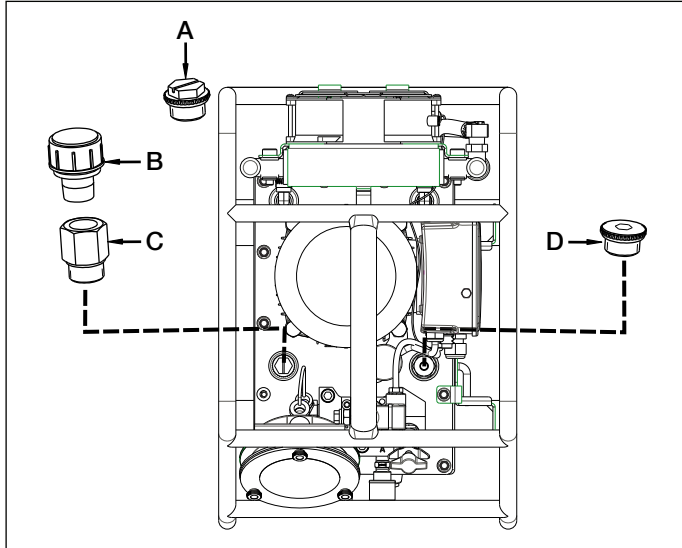
Figuur 1, Reservoir ontluichtingsdop en olievuldop
