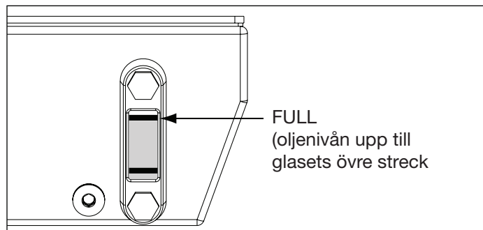
Figur 2, Inspektionsglas
