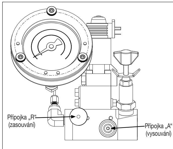
Obrázek 4, Připojky ventilu
