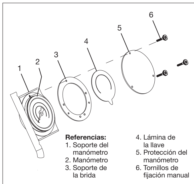
Figura 9, Lámina del manómetro
