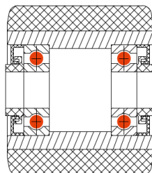
Labyrinthabdichtung
