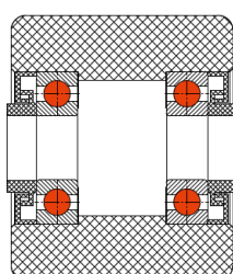
Labyrinthabdichtung
