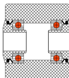
V-Ring-Abdichtung
