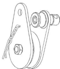
Puleggia EH/EGZ
