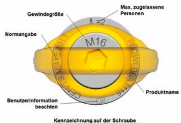
Bild 3: Teilebezeichnung und Ort der Identifizierungsdetails am Produkt
