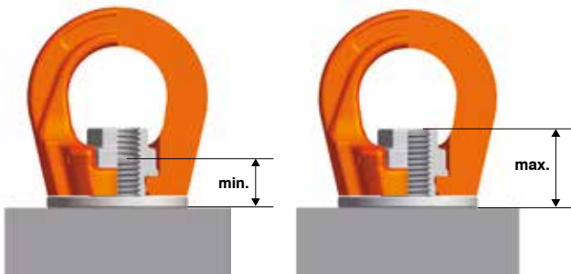
Bild 6: Einschraublänge Minimum
