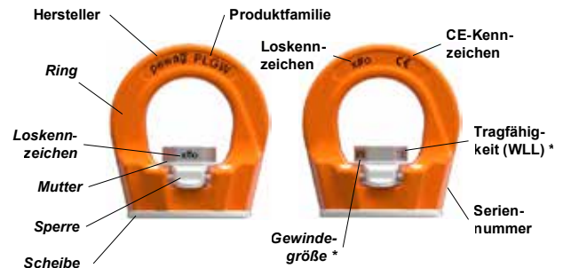
Bild 3: Teilebezeichnung und Ort der Identifizierungsdetails am Produkt
