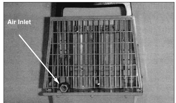
図4-PAMポンプのエア入口ポート
