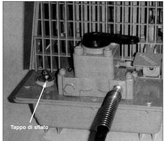
Figura 2 - Posizione del tappo di sfiato/riempimento del serbatoio
