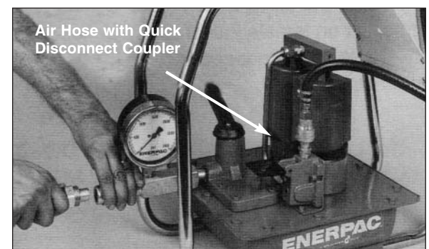
図5-EAMポンプのエア入口ポート
