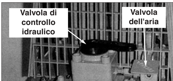
Figura 6 - Controlli pompa
